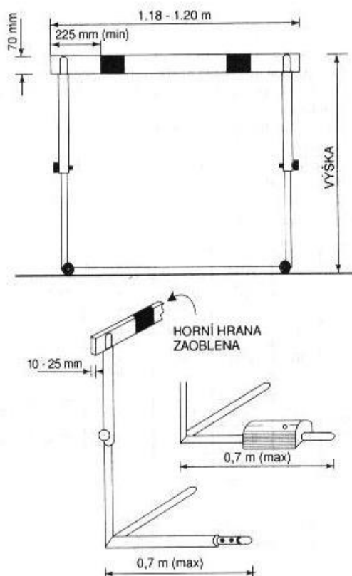
Obr. 168 - příklad provedení překážky
