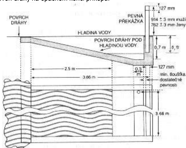
Obr. 169b - vodní příkop
