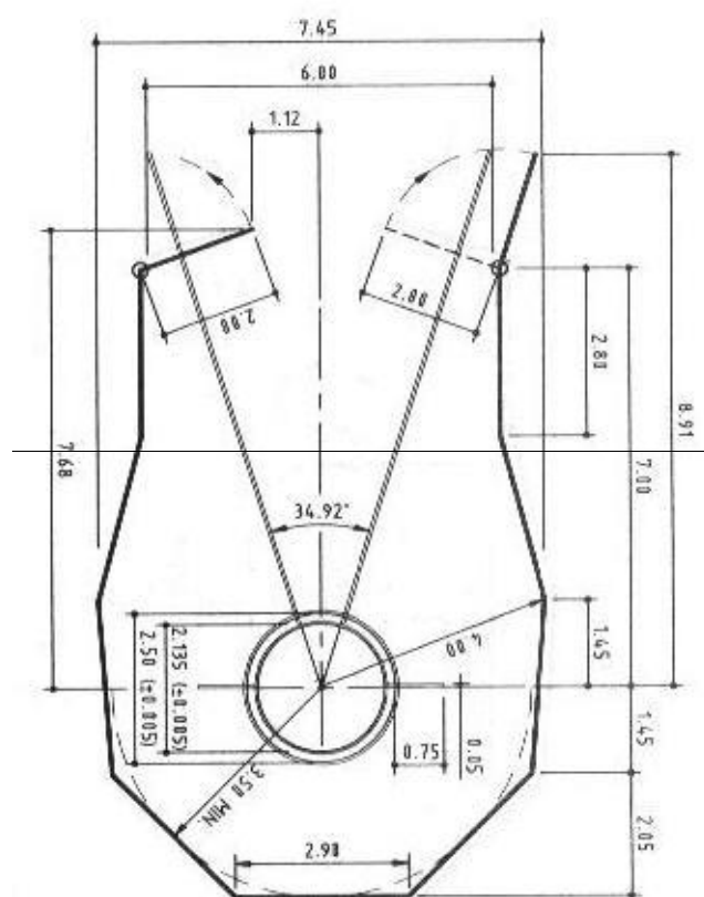
Obr. 192a - Klec se soustřednými kruhy pro hody diskem a kladivem nastavená pro hod kladivem
