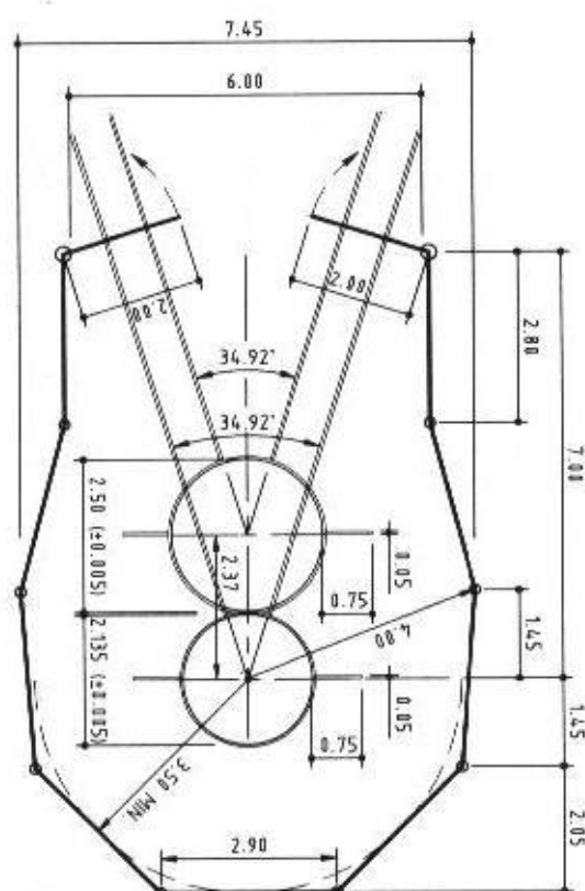
Obr. 192c - Klec se samostatnými kruhy pro hody diskem a kladivem nastavená pro hod kladivem
