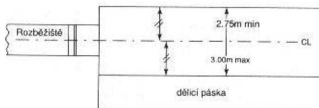
Obr. 184b - Doskočiště pro skok do dálky a trojskok
