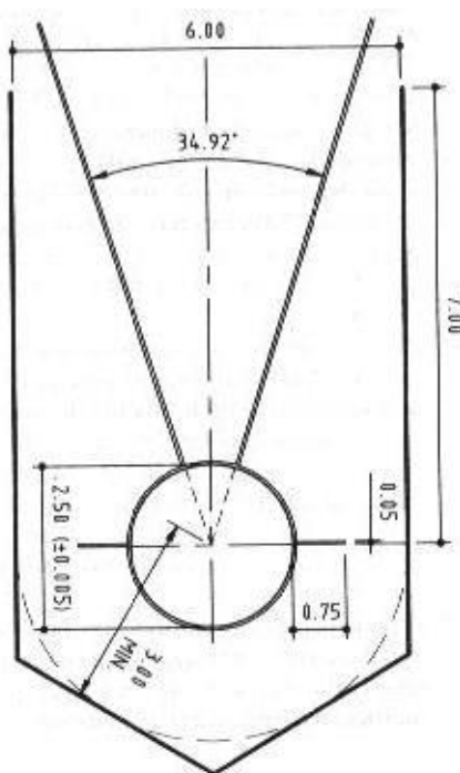
Obr. 190 - klec pro hod diskem
