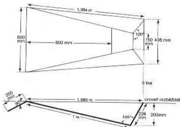
Obr. 183a - Skříňka pro skok o tyči
