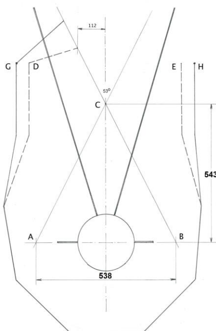
Obr. 192d – Stanovení úhlu největšího ohrožení (zóny ohrožení).
